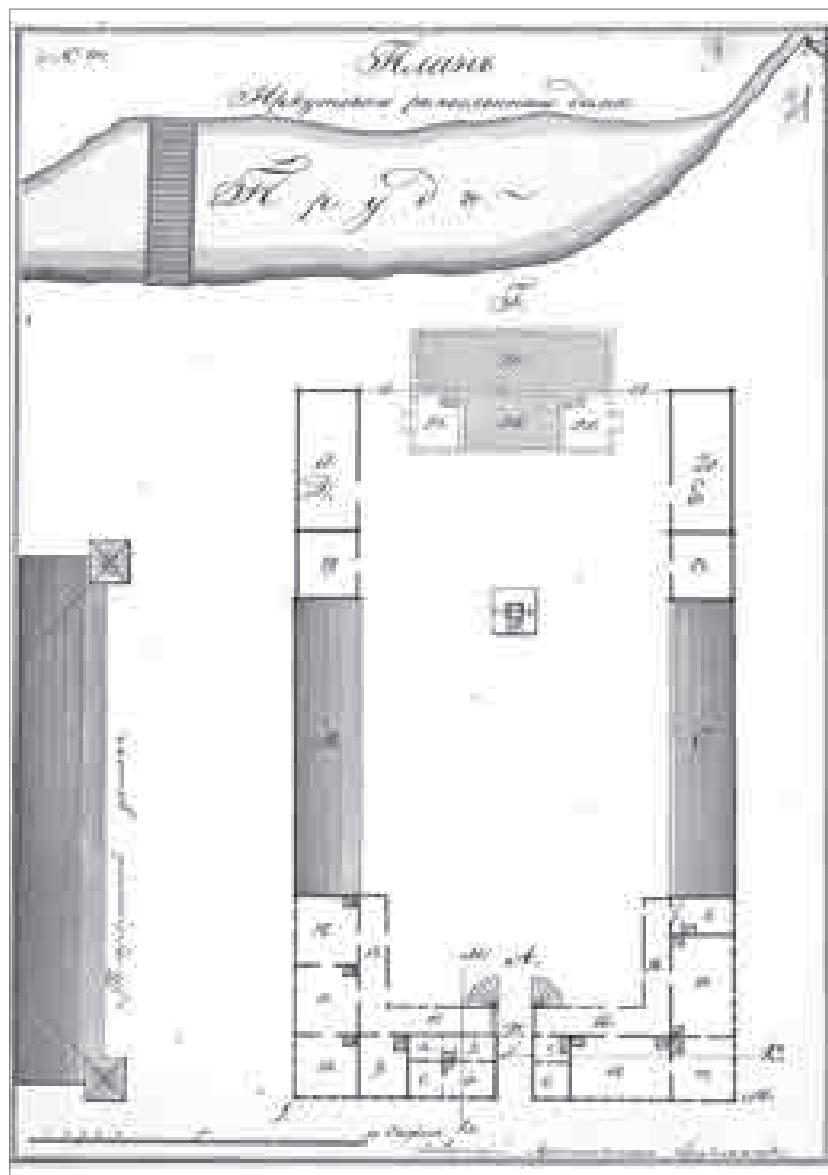
План Иркутского ремесленного дома. РГИА. Публикуется впервые
