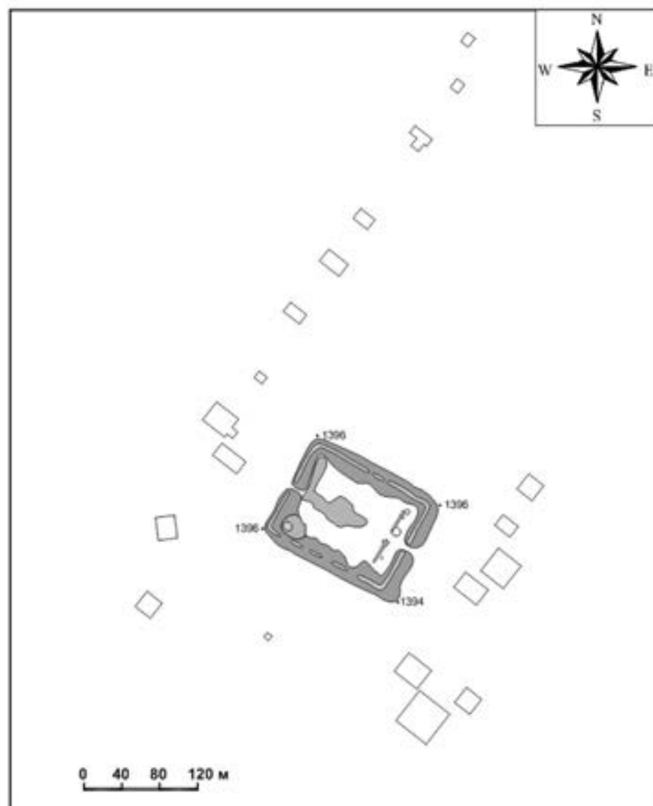
Рис. 7. План городища Сангян ширээтийн балгас. Монголия, Центральный аймак, 2012 г.
