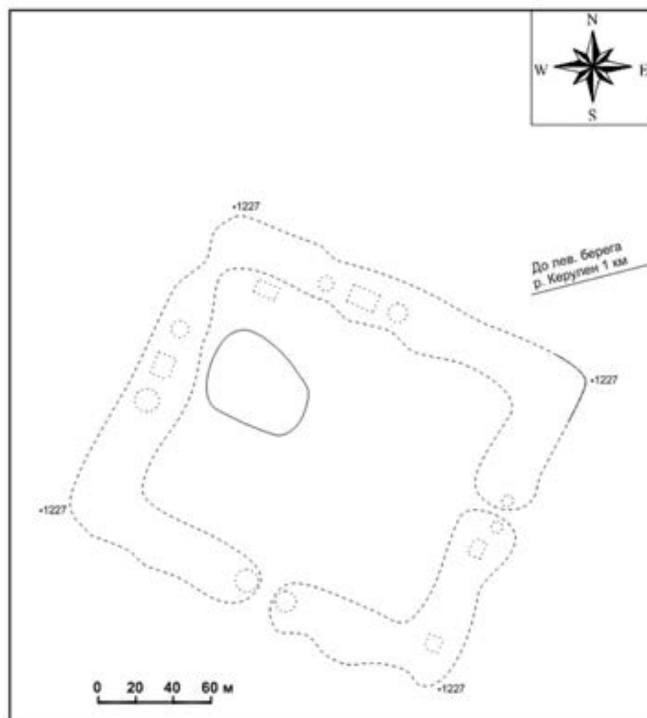
Рис. 2. План городища Гуа дов. Монголия, Центральный аймак, 2011 г.
