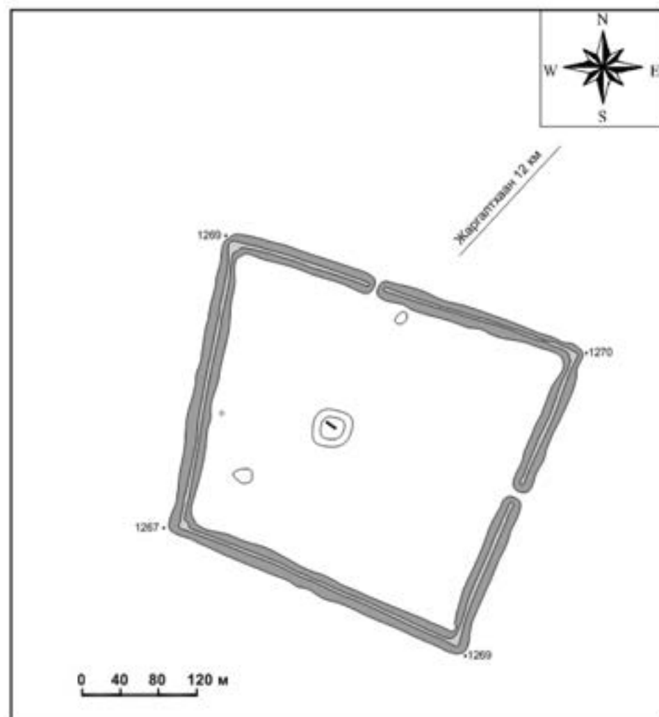
Рис. 6. План городища Цикхэрийн голын хэрэм. Монголия, Хэнтийский аймак, 2011 г.
