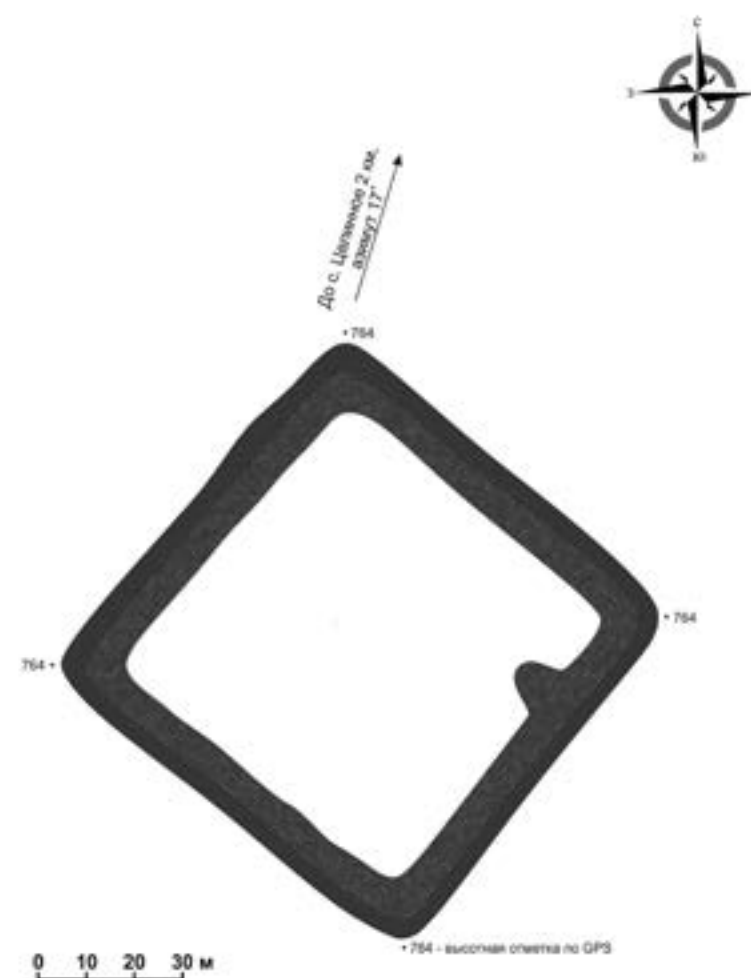
Рис. 3. Городище Кыйлыг-Хову (Целинное), план
